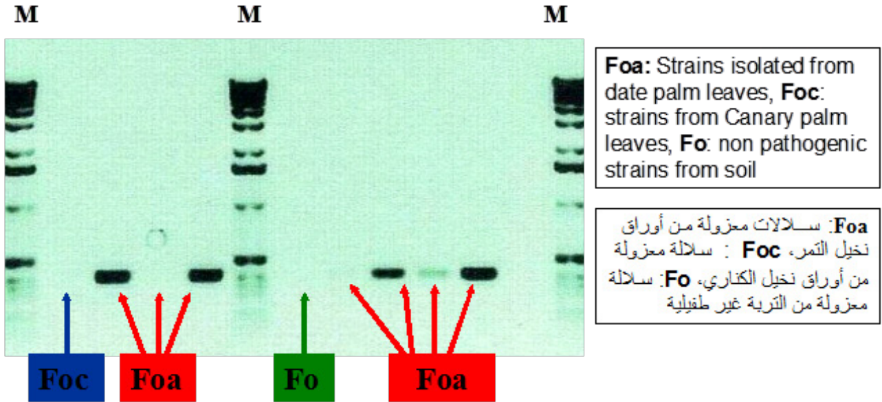
رسم 6. نتائج تكثيف أجزاء الحمض النووي لسلالات الفطر المسبب لمرض البيوض مأخوذة من نخيل غير ممرضة باستخدام زوج من المبدئيات (TL3 و Foa 28) وتقانة التكثيف المختص. M: شاهد عن وزن أجزاء الحمض. (Foa28: ATCCCCGTAAAGCCCTGAAGC، TL3: GGTCGTCCGAGAGTATACCGGC) Molecular profile of Specific PCR-DNA products of some pathogenic strains on date and Canary palms and non pathogenic strains from soil revealed by two primers (TL3 and Foa 28). M: molecular weight marker
