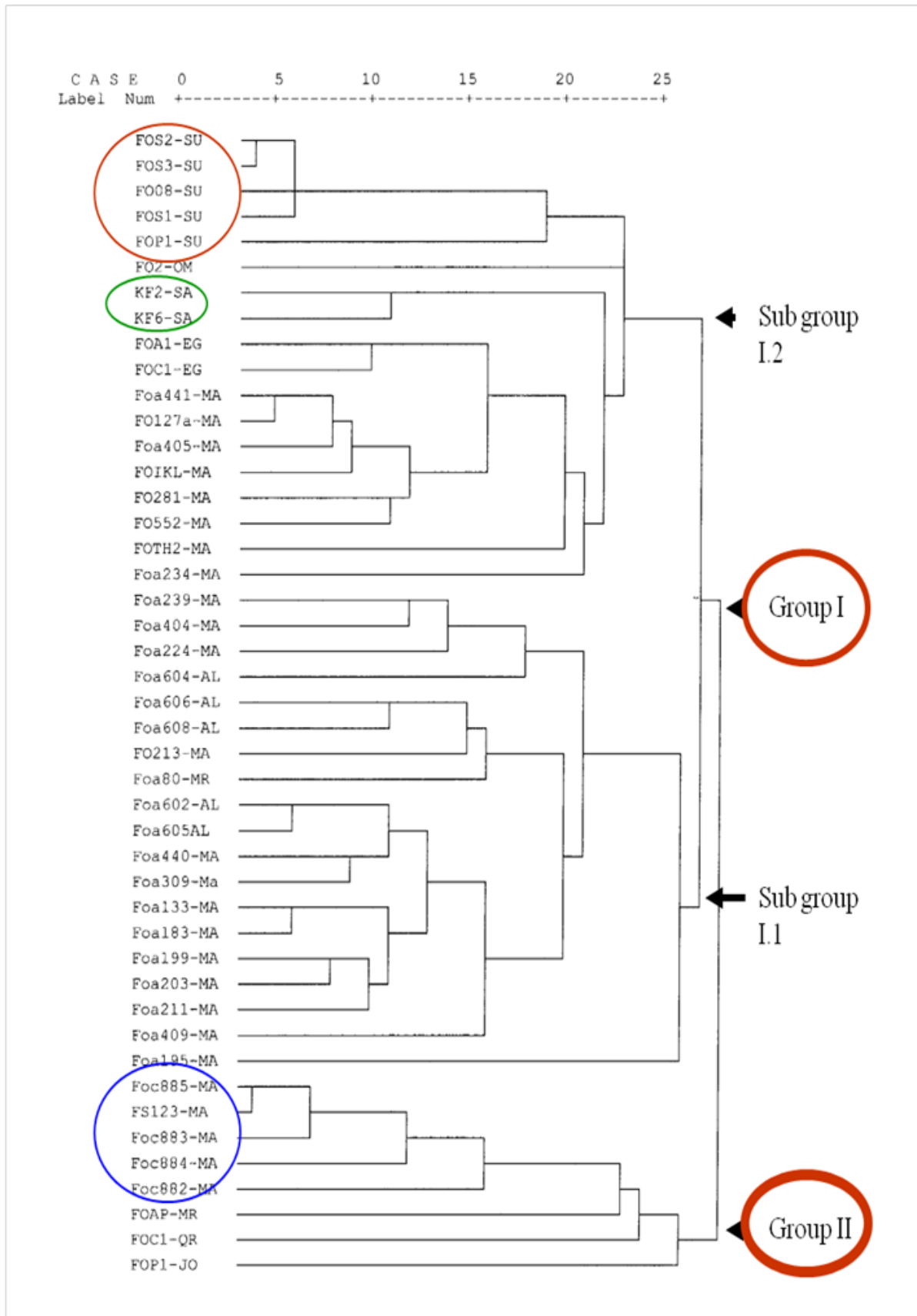
رسم 8. تجمع وتقارب وتباعد السلالات الطفيلية وغير الطفيلية حسب أصولها ومواقعها الجغرافية باستخدام تقانة ISSR على 45 سلالة من المغرب و من أصول مختلفة من الدول العربية.
